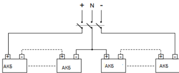
Рис. 3-11 Схема подключения аккумуляторных цепочек
