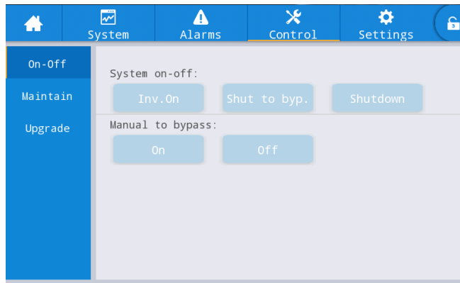
Рис. 4-18 Интерфейс включения-выключения
