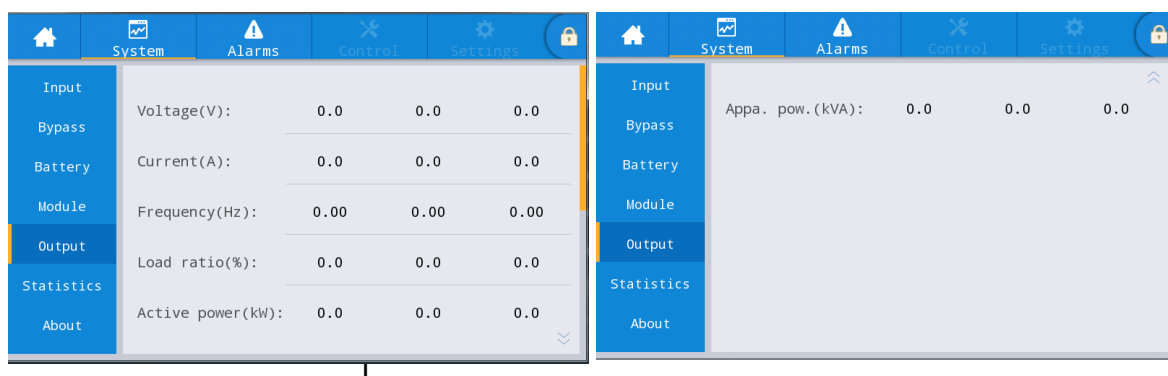
Рис. 4-12 Интерфейс меню выходных параметров
