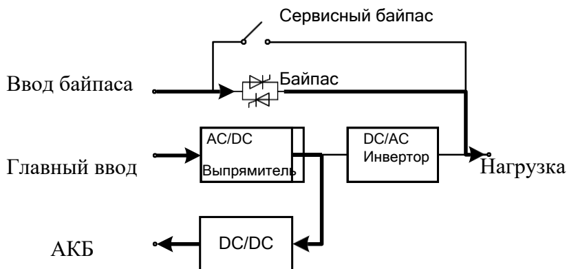
Рис. 2-5 Принцип работы режима ЕСО
