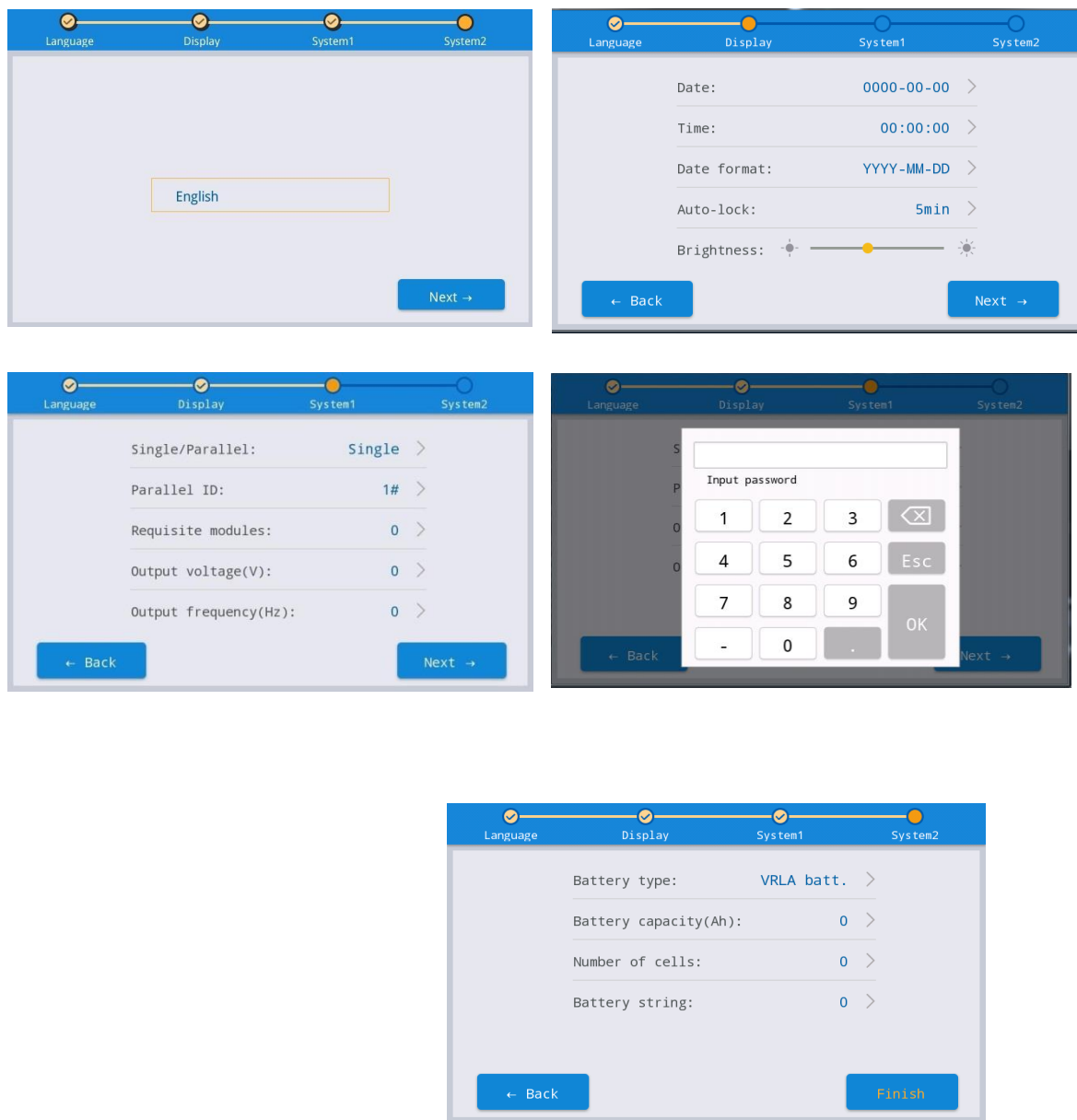
Рис. 4-3 Быстрые настройки
