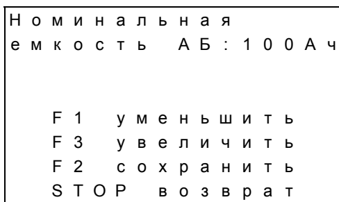
Рис.33. Номинальная емкость АБ
