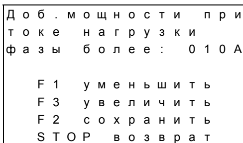
Рис.39 Порог добавления мощности
