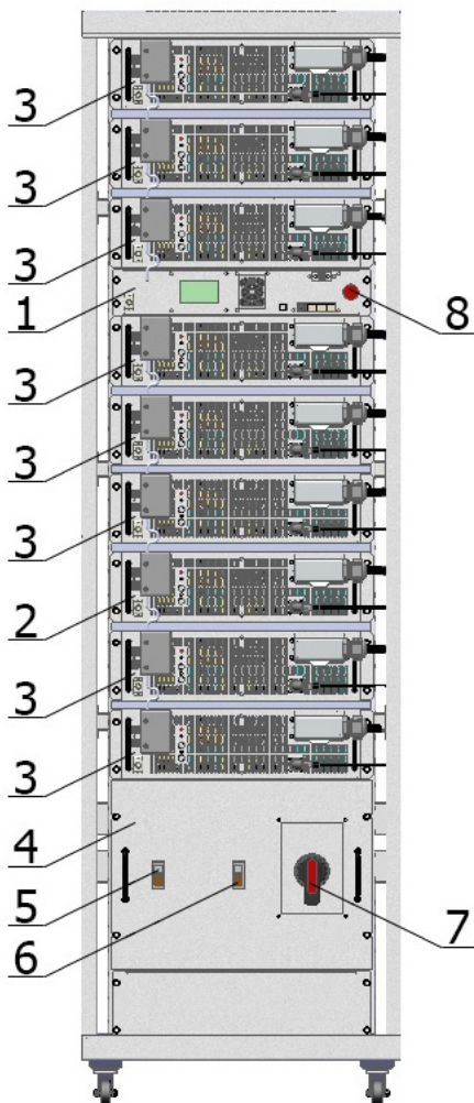
Рис. 1 ИБП RUPO-3-90К. Вид спереди.
