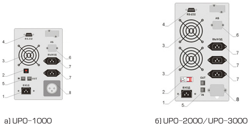
Рис. 2. Задняя панель блока ИБП:
